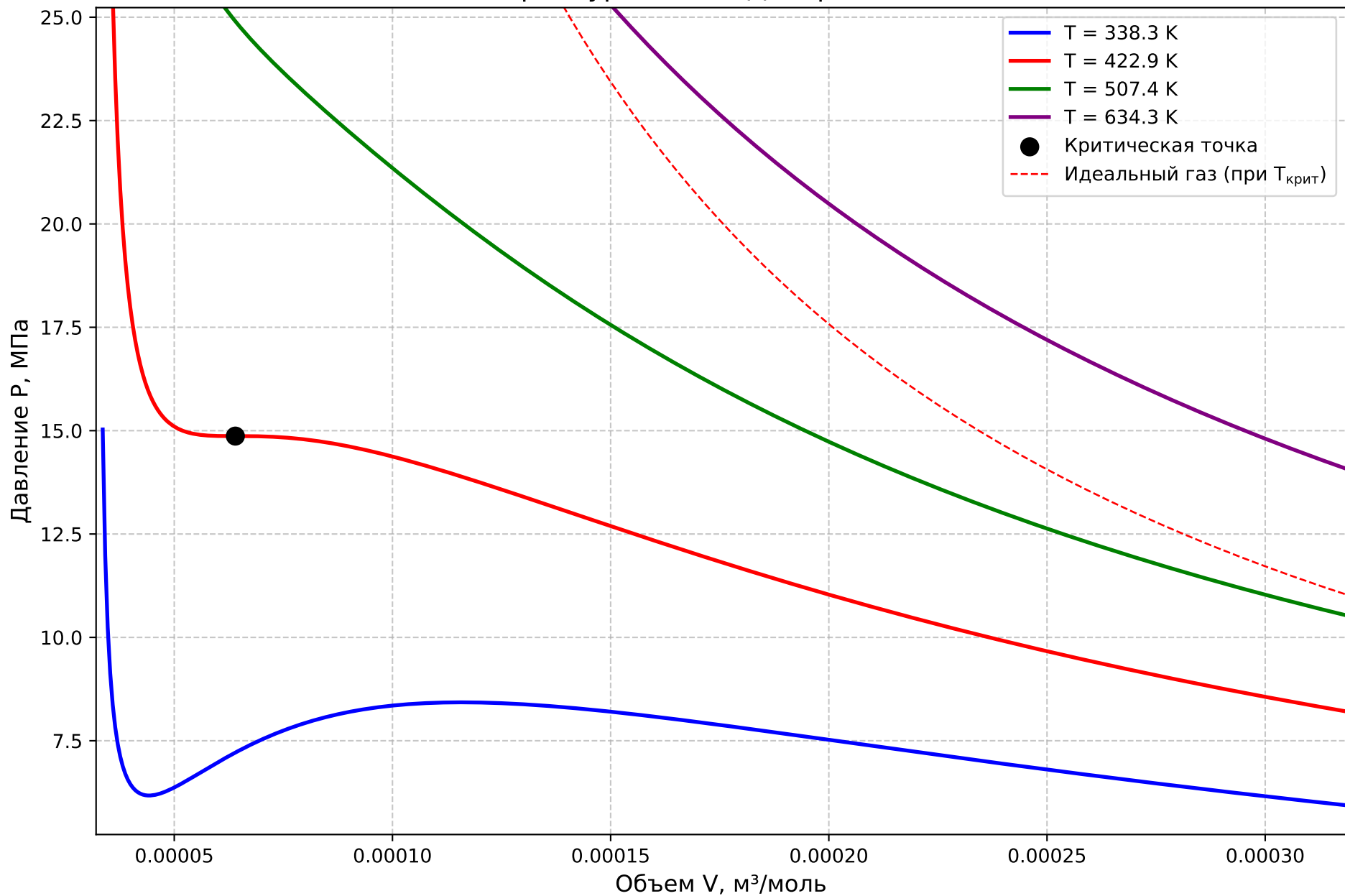
Изотермы уравнения Дитеричи для \text{CO}_2
